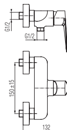
Bateria natryskowa ścienna
