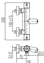
Bateria wannowa termostatyczna
