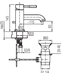
Bateria umywalkowa
