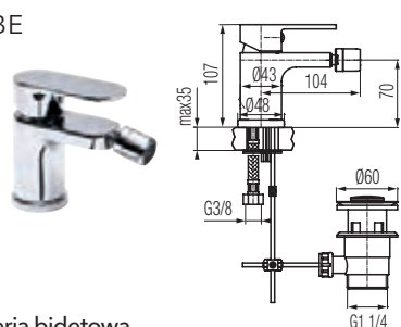
Bateria bidetowa
