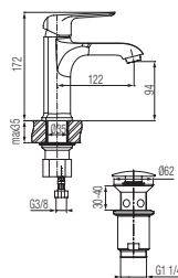
Bateria umywalkowa wysoka
