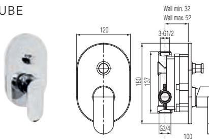
Bateria wannowo-natryskowa podtynkowa
