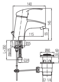
Bateria umywalkowa
