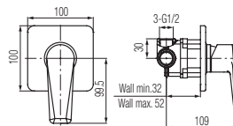
Bateria natryskowa podtynkowa
