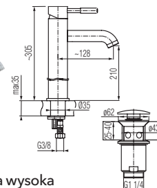
Bateria umywalkowa wysoka
