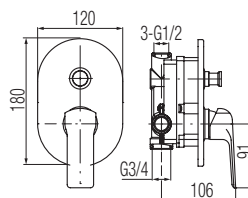
Bateria wannowo-natryskowa podtynkowa
