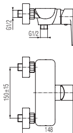
Bateria natryskowa ścienna
