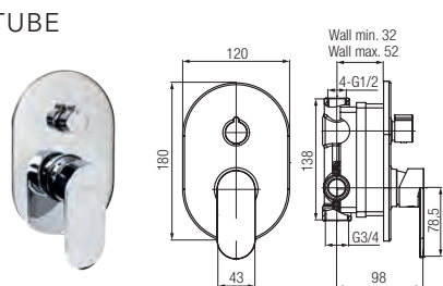
Bateria podtynkowa 3-funkcyjna
