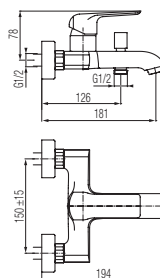
Bateria wannowa ścienna
