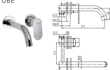
Bateria umywalkowa podtynkowa
