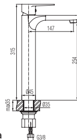
Bateria umywalkowa wysoka
