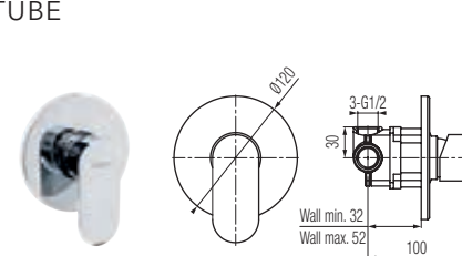
Bateria natryskowa podtynkowa
