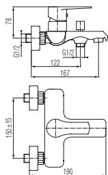
Bateria wannowa ścienna
