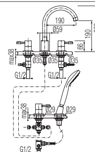
Bateria wannowa 5-otworowa
