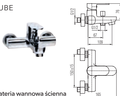
Bateria wannowa ścienna
