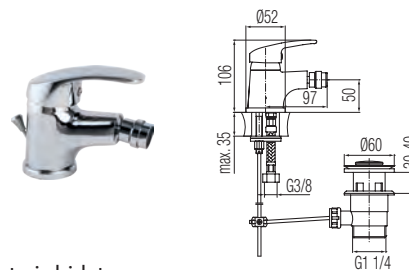
Bateria bidetowa
