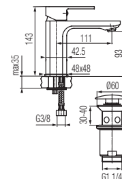
Bateria umywalkowa
