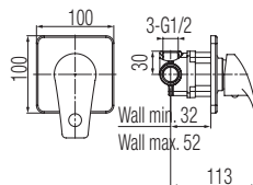
Bateria natryskowa podtynkowa
