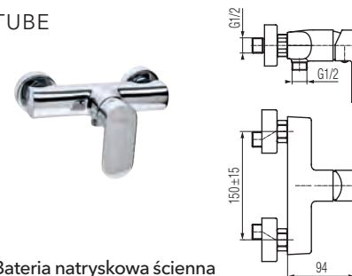
Bateria natryskowa ścienna
