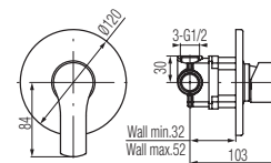
Bateria natryskowa podtynkowa
