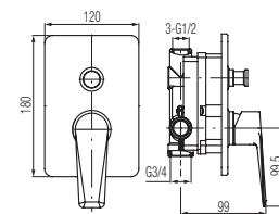
Bateria wannowo-natryskowa podtynkowa
