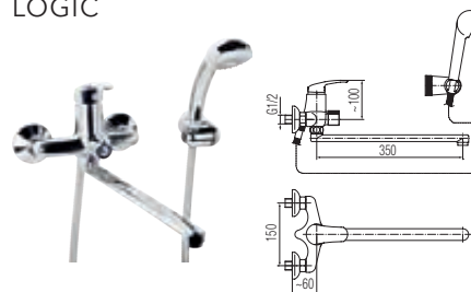
Bateria wannowo-umywalkowa ścienna
