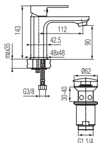
Bateria umywalkowa
