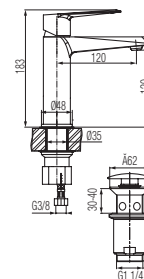
Bateria umywalkowa
