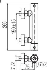
Bateria natryskowa termostatyczna
