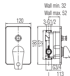
Bateria wannowo-natryskowa podtynkowa
