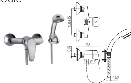
Bateria natryskowa ścienna
