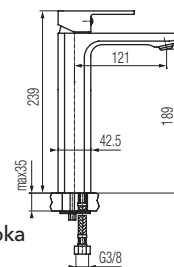
Bateria umywalkowa wysoka (270 mm)
