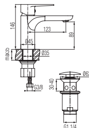
Bateria umywalkowa wysoka
