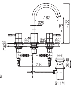
Bateria umywalkowa 3-otworowa
