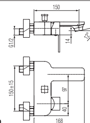
Bateria wannowa ścienna
