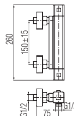
Bateria natryskowa termostatyczna
