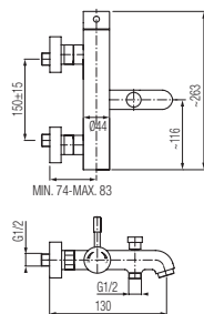
Bateria wannowa ścienna
