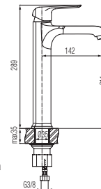
Bateria umywalkowa wysoka
