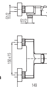
Bateria natryskowa ścienna
